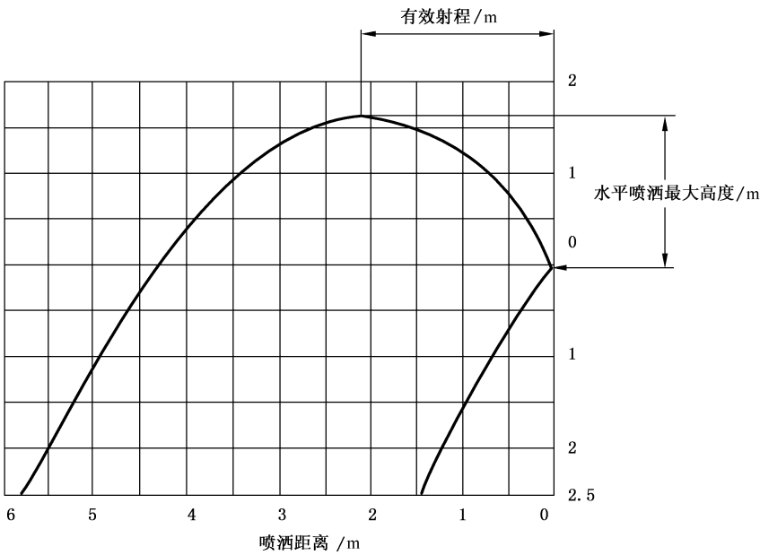
图 B.2 水平喷洒图
