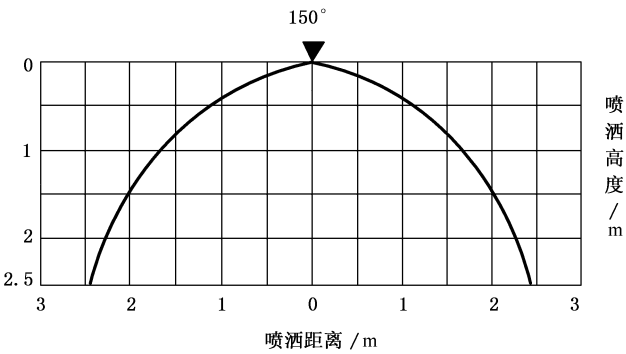
图 B.1 垂直喷洒图
