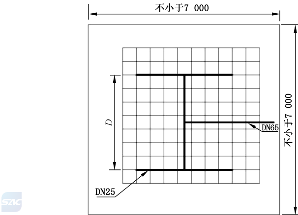
图 1 布水试验管路布置图
