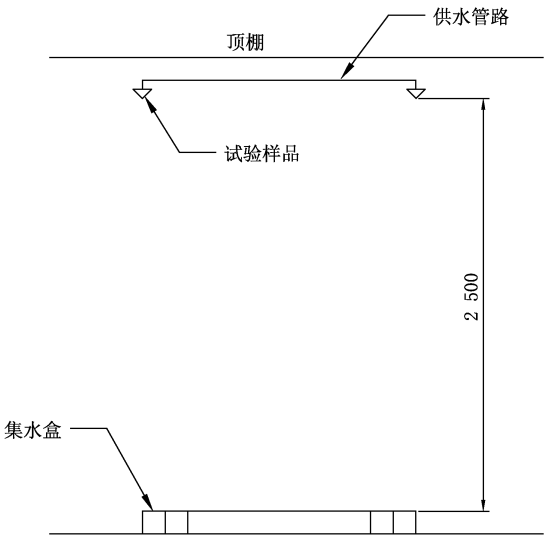
图 2 布水试验侧视图
